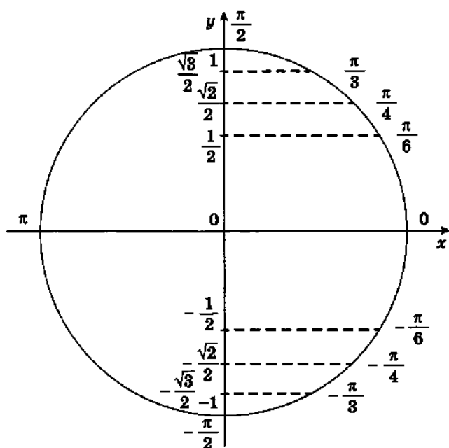
Рис. 4. Линия синусов
