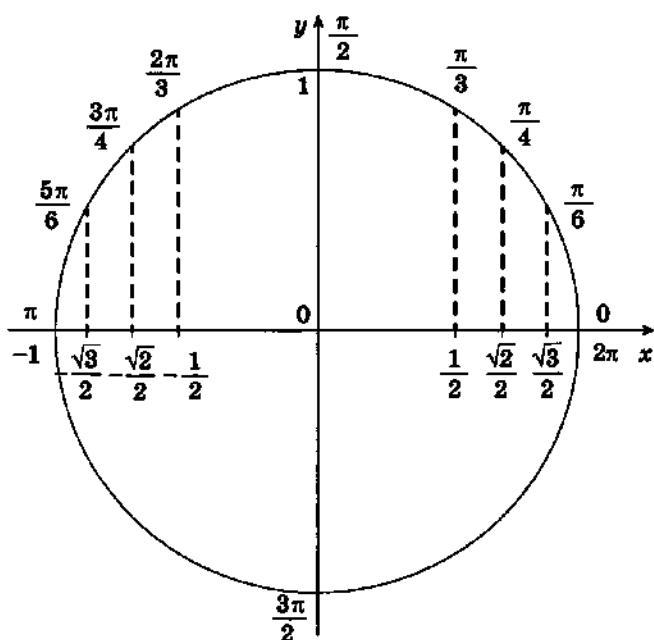
Рис. 5. Линия косинусов
