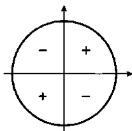
Знаки тангенса
