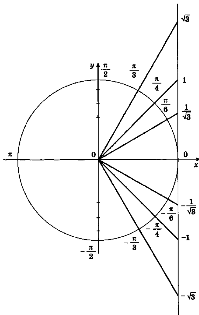
Рис. 6. Линия тангенсов
