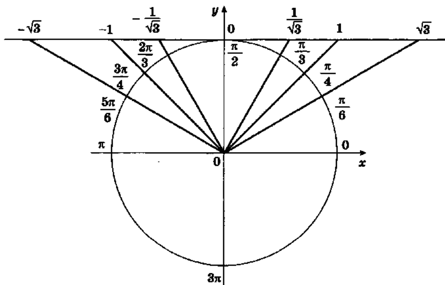
Рис. 7. Линия котангенсов
