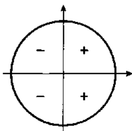
Знаки косинуса
